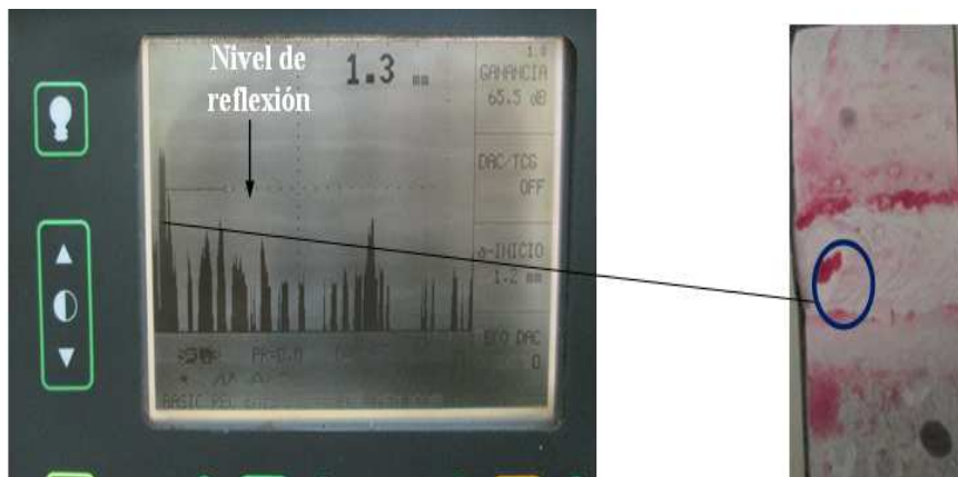
Figura 3.10. Resultados obtenidos para el electrodo UTP 65.
