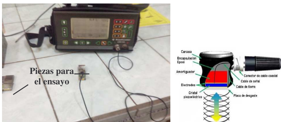
Figura 2.8. Equipo de ultrasonido y esquema del palpador ultrasónico empleados.
