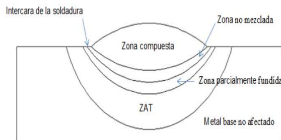
Figura 1.5. Zonas de la unión soldada. Fuente: Marulanda et al. (2007b).
