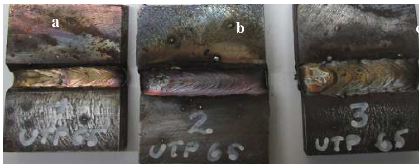
Figura 2.3. Muestras soldadas con electrodos UTP 65.
