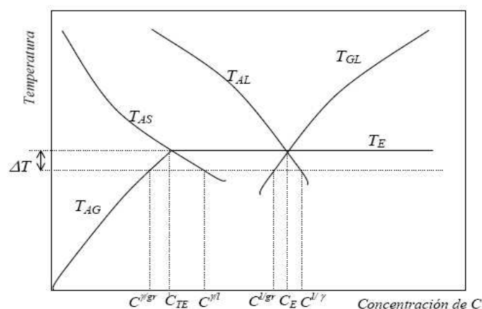
Figura 2.2. Región eutéctica del diagrama un Fe-C-Si para un determinado porcentaje de Si.
