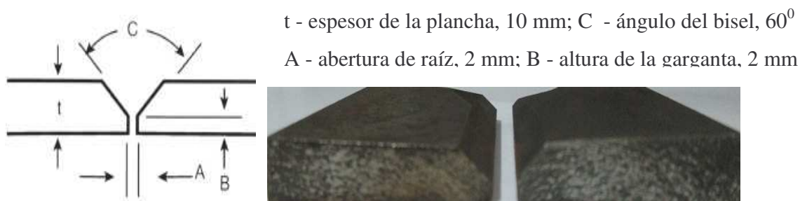
Figura 2.5. Preparación de la junta en las muestras para la soldadura
