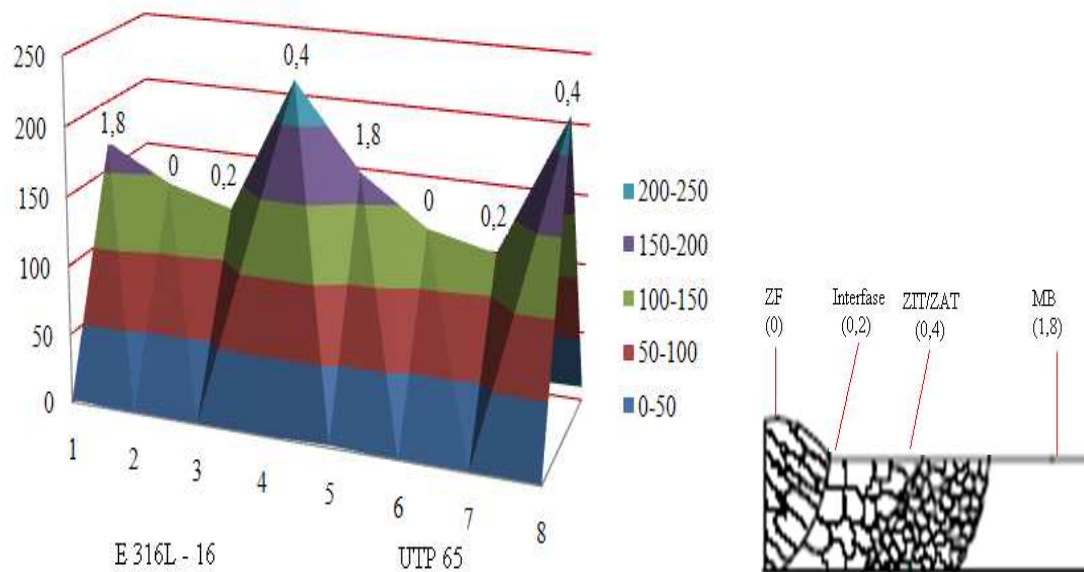
Figura 3.8. Comportamiento de la dureza para diferentes distancia en las diferentes zonas.
