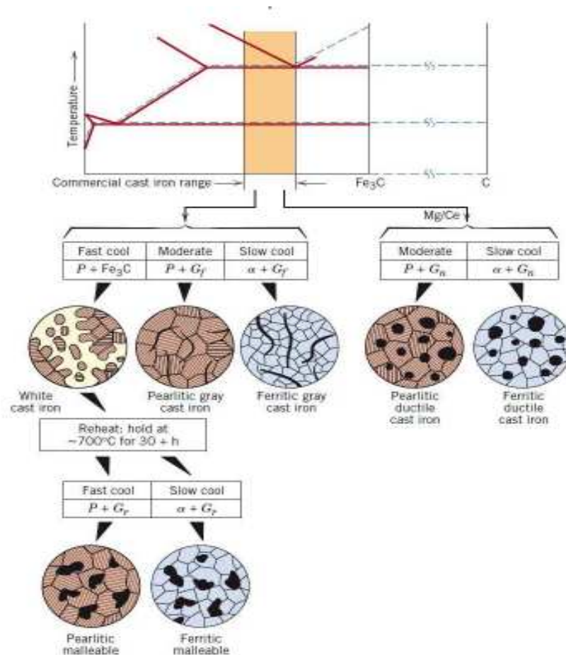
Figura 1.3. Variedad de microestructuras según la variación de temperatura.
