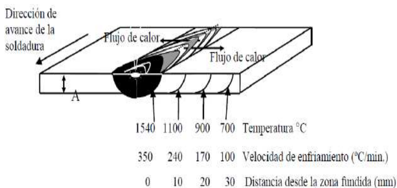
Figura 1.4. Distribución de temperatura y velocidad de enfriamiento.
