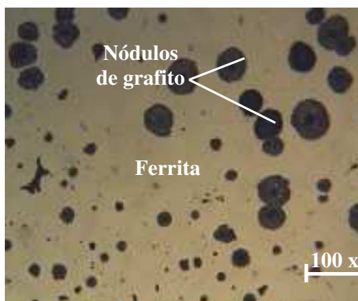
Figura 1.2. Microestructura del hierro nodular. Fuente: Apraiz (1963).
