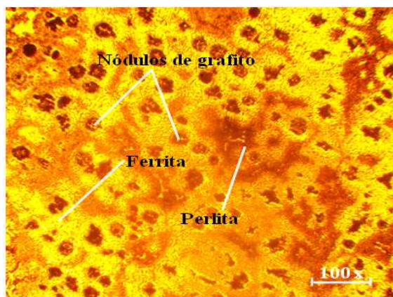
Figura 2.2. Microestructura del hierro fundido nodular.
